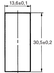
Монтажный вырез
